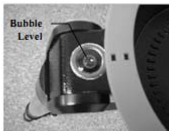
Obrázek 2.2 - vodováha
