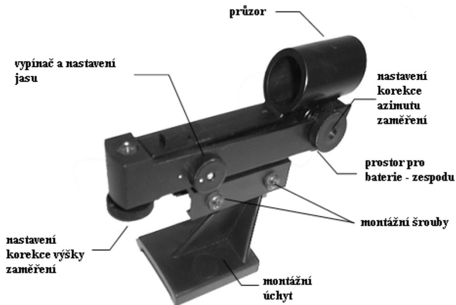
Obrázek 2.7 – Popis hledáčku StarPointer
